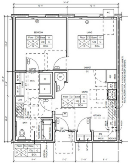
Unit 1B1-A Type: K 650 SF - 1.74US
