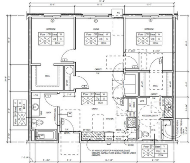
Unit 2B1-A Type: K 935 SF - 1.74US
